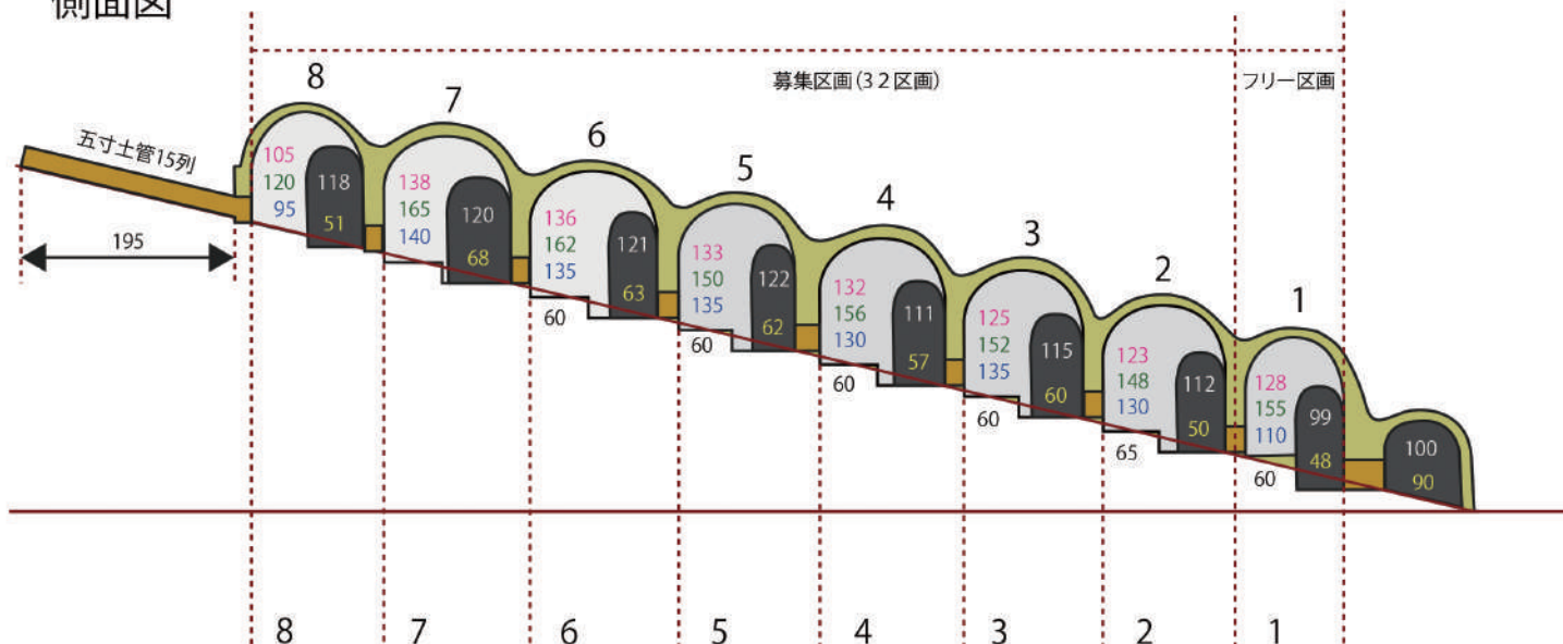
側面図
